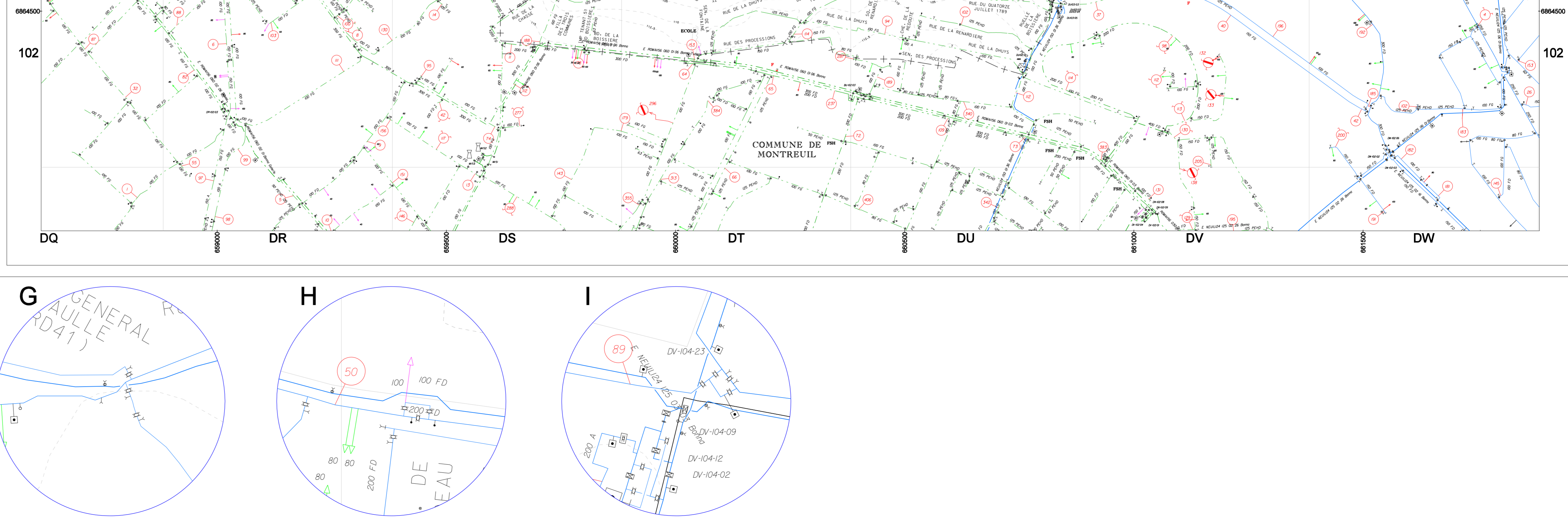
6.2.2 Les réseaux d'eau potable, d'assainissement eaux usées et eaux pluviales : Plan du réseau EAU PLU Ville de Noisy-le-Sec PIÈCE 6 - 6.2 Annexes sanitaires
